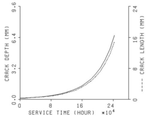
20 pav. Įtempties korozijos defekto raida, kai T min = 5,08 mm
