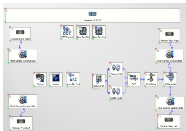
2 pav. „Maserati MC20“, AVL CRUISE modelis Šaltinis: sudaryta autoriu
