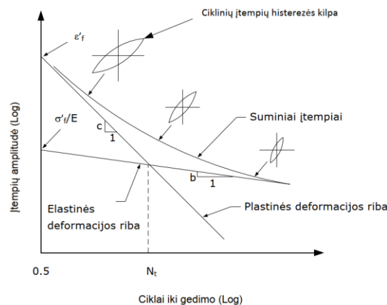
1 pav. S-N kreivė Šaltinis: API 579, 2021
